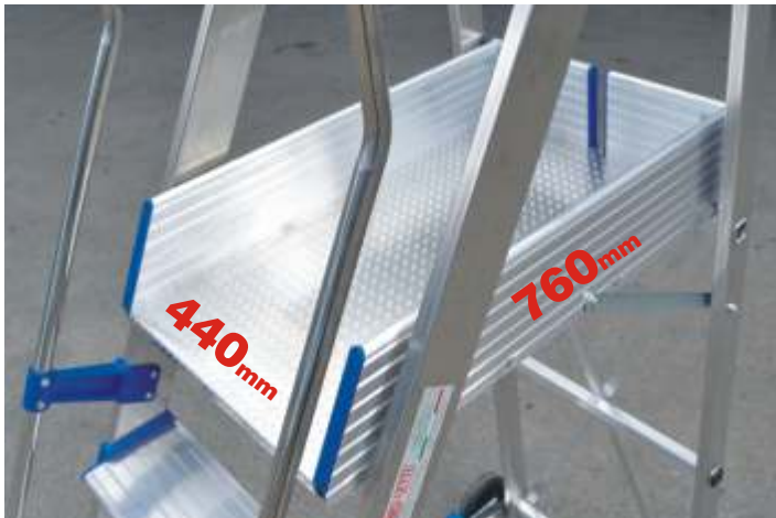
Piattaforma di lavoro mm 760x440 in lamiera mandrolata di alluminio con tavole fermapiede Workplatform 760x440 mm in grooved aluminum sheet, with toaboards
